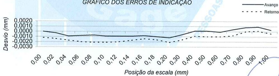
GRÁFICO DOS ERROS DE INDICAÇÃO
